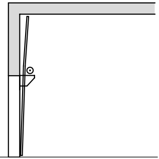
Prowadzenie VU z obniżonym wałem sprężyny skrętej
