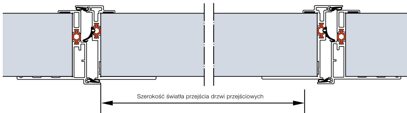
Konstrukcja drzwi przejściowych z przegrodą termiczną w bramach segmentowych o grubości konstrukcji 67 mm
