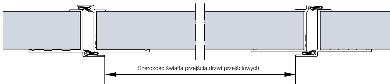
Konstrukcja drzwi przejściowych w bramach segmentowych o grubości konstrukcji 42 mm
