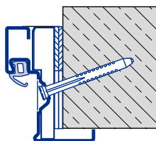
Ościeżnica kątowna Mocowanie diagonalne A Typ 1
