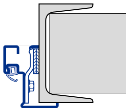
Ościeznica kątowa, montaż przez spawanie A Typ 3
