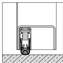
Opadająca uszczelka progowa, hydrauliczna, z opóóznieniem opadania, typ A2
