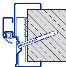
Ościeżnica kątowna z ościeżnicą uzupełniającą Vario B53 Mocowanie diagonalne C Typ 1
