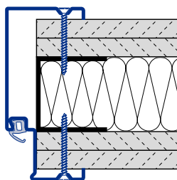
Ościeznica obejmująca B73 do ścian kartonowo-gipsowych Montaż przez skręcanie C Typ 4
