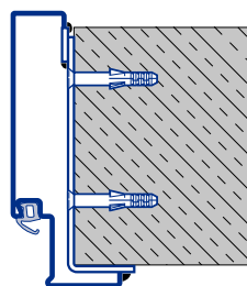
Ościeżnica obejmująca Montaż na kołki rozporowe przez spawanie D Typ 1
