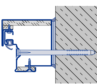
Ościeznica blokowa 2-częściowa Montaż na kołki rozporowe przez ościeże E Typ 2
