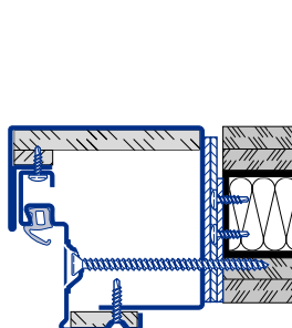
Ościeznica blokowa 2-częściowa Montaż na kołki rozporowe przez ościeże E Typ 2
