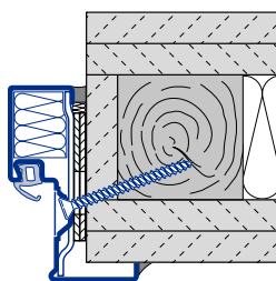
Ościeznica DryFix Mocowanie diagonalne B Typ 1
