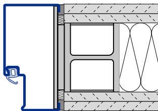
Ościeznica blokowa, montaż przez spawanie E Typ 1
