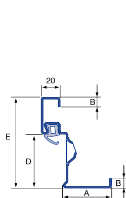
Ościeżnica kątowna Mocowanie diagonalne
