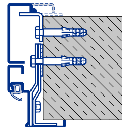
Ościeżnica kątowna i uzupełniająca Montaż na kołki rozporowe C Typ 3
