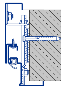
Ościeżnica obejmująca 2-częściowa Lico ościeżnicy 33 mm D Typ 3
