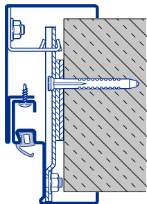
Ościeżnica obejmująca 2-częściowa Lico ościeżnicy 76 mm D Typ 3
