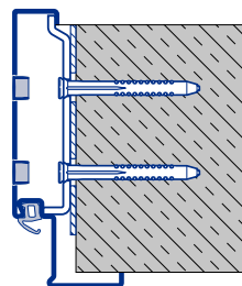
Ościeżnica obejmująca Montaż na kołki rozporowe przez ościeże od szerokości obejmy 205 mm D Typ 1
