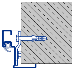
Ościeżnica kątowna Montaż na kołki rozporowe niewidoczny A Typ 2
