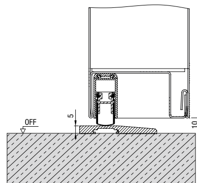
3 z uszczelką i progiem
