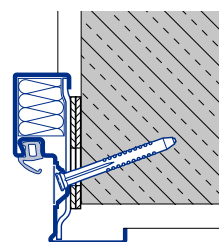
Ościeznica DryFix Mocowanie diagonalne B Typ 1
