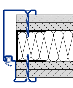
Ościeznica obejmująca B73 do ścian kartonowo-gipsowych Montaż przez skręcanie C Typ 4
