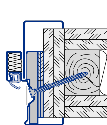
Ościeznica kątowa z ościeznicą uzupełniającą Vario B53 Mocowanie diagonalne C Typ 1
