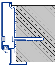
Ościeżnica obejmująca Montaż na kołki rozporowe przez ościeże do maksymalnej szerokości obejmy 204 mm D Typ 1
