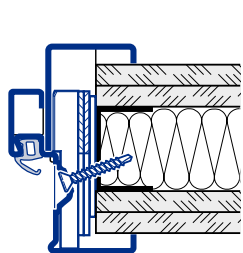
Uniwersalna ościeznica kątowa z ościeznicą uzupełniającą Vario B53 Mocowanie diagonalne C Typ 1
