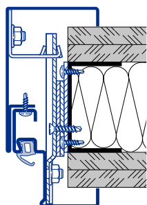
Ościeznica obejmująca 2-częściowa (Lico ościeznicy 76 mm) Ściany kartonowo-gipsowe F90 A D Typ 3
