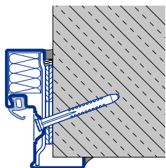
Ościeżnica DryFix Mocowanie diagonalne B Typ 1
