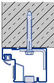
Ościeznica blokowa do montażu przed ścianą E Typ 3
