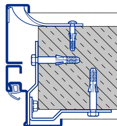
Ościeznica kątowna z ościeźnicą uzupełniającą Montaż na kołki rozporowe C Typ 3
