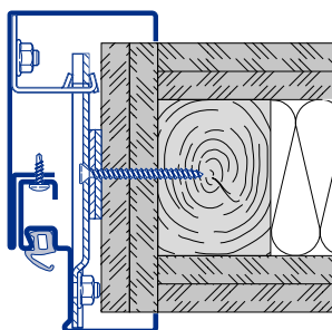
Ościeznica obejmująca 2-częściowa (Lico ościeznicy 76 mm) Ściany kartonowo-gipsowe F90 B D Typ 3
