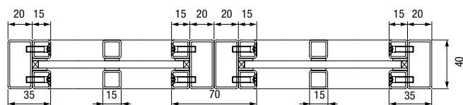
Przekrój poziomy
