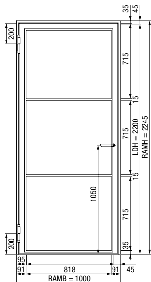
1-skrzydłowe drzwi rozwierne
