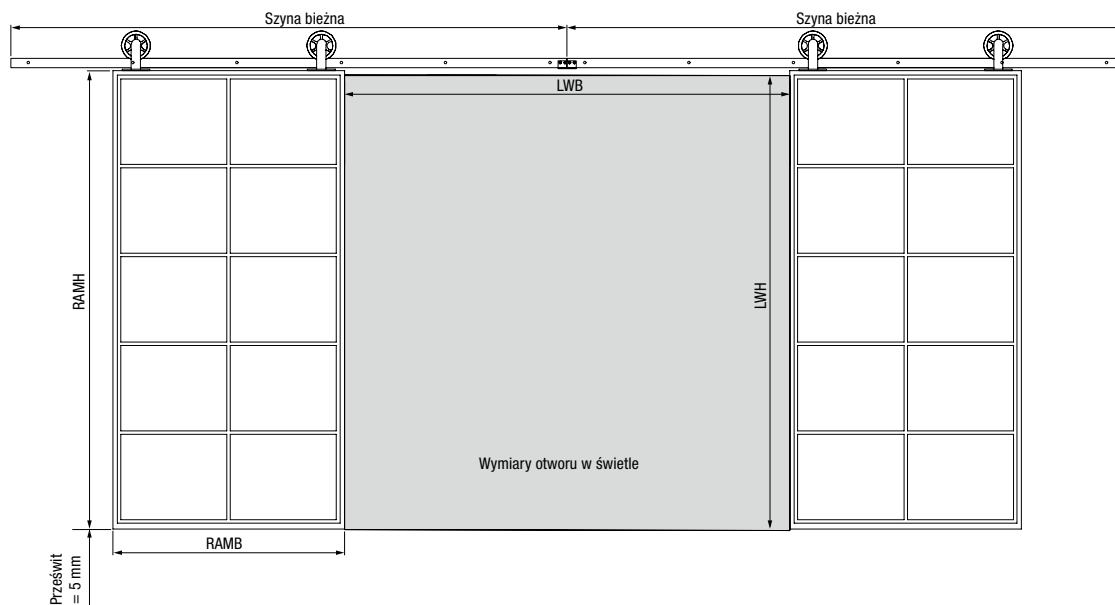
2-skrzydłowe drzwi przesuwne Retro Loft
