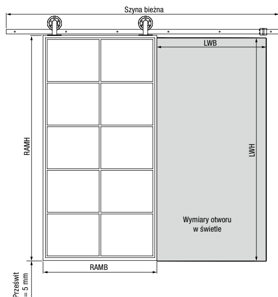
1-skrzydłowe drzwi przesuwne Retro Loft
