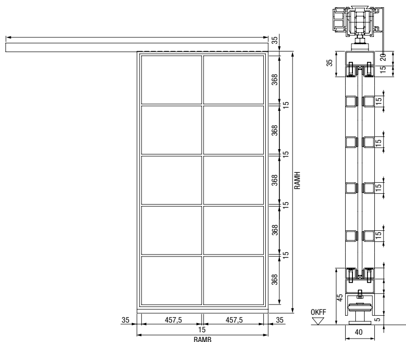
1-skrzydłowe drzwi przesuwne
