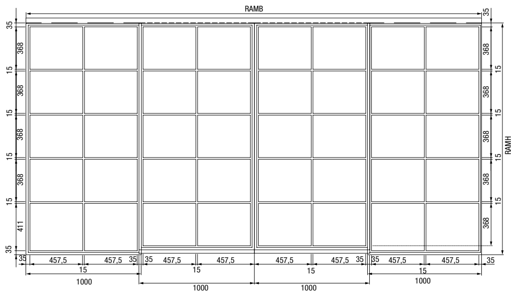
2-skrzydłowe drzwi przesuwne z naświetlami bocznymi
