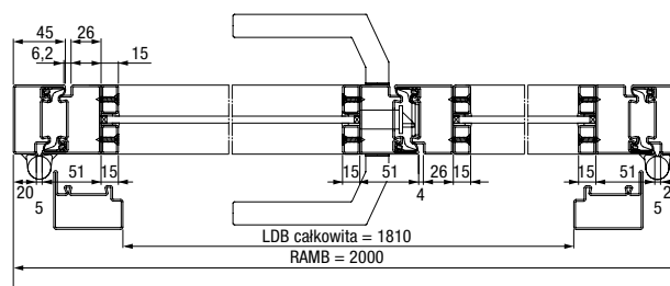
2-skrzydłowe drzwi rozwierne, przekrój poziomy
