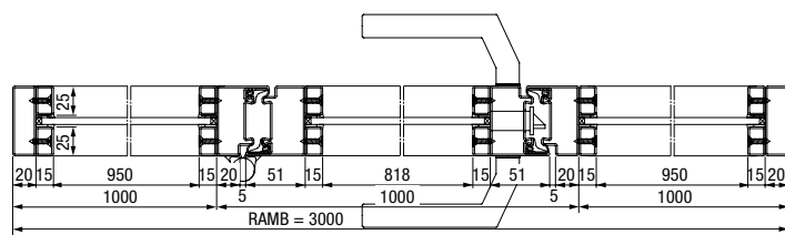
Przekrój poziomy
