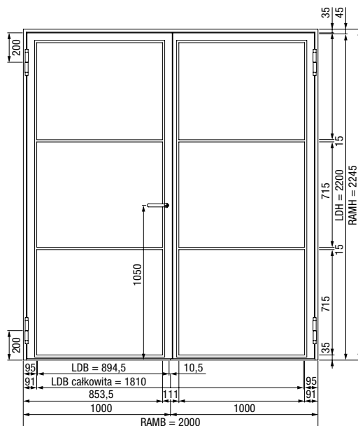
2-skrzydłowe drzwi rozwierne
