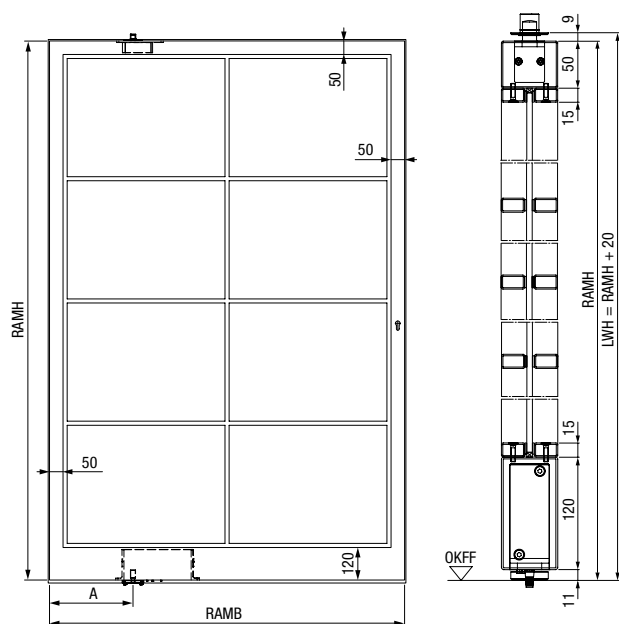
Drzwi Pivot z profilem ramy o szerokości 50 mm i cokółem o wysokości 120 mm, symetryczny układ szpros
