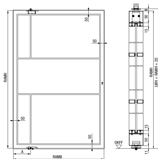
Drzwi Pivot w standardowej wersji wykonania z profilem ramy o szerokości 50 mm i cokółem o wysokości 50 mm, wzór 1
