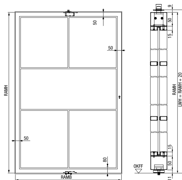
Drzwi Pivot w standardowej wersji wykonania z profilem ramy o szerokości 50 mm i cokółem o wysokości 50 mm, wzór 2
