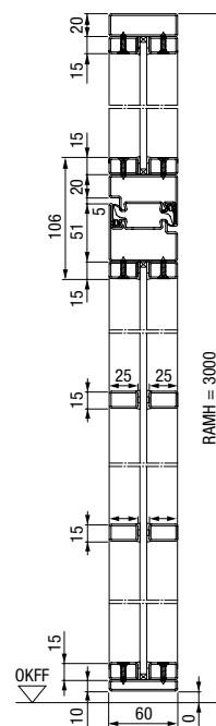
Przekrój pionowy
