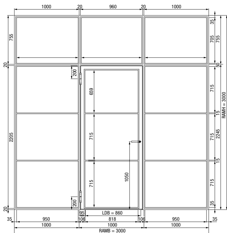
1-skrzydłowe drzwi rozwiernie z naświetlami bocznymi i naświetlem górnym
