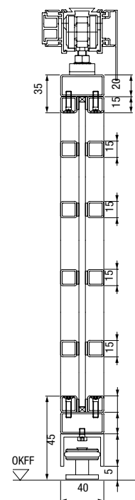
Przekrój pionowy
