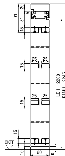
Przekrój pionowy
